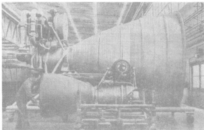
图 3.7 F-1 型发动机的外形 (里面的 F-1 的原尺寸模型,外面的是 H-1 发动机)
