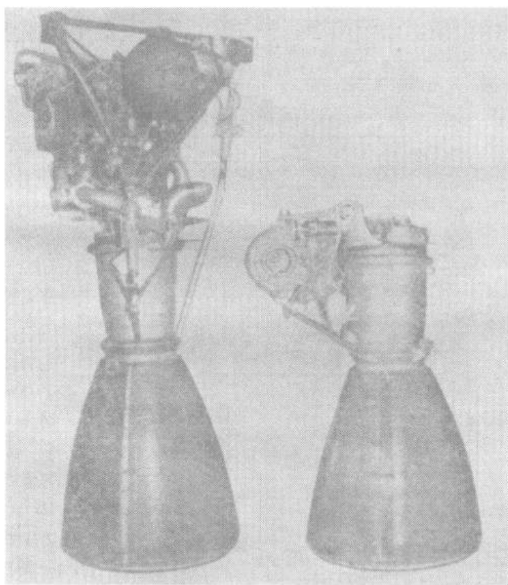
图 3.4 86 吨推力发动机的外形
