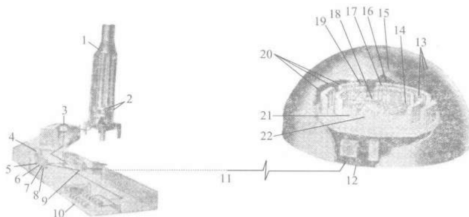
图 4.12 “土星”火箭发射操纵室
