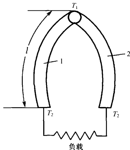
图 13.11 热电偶电路
