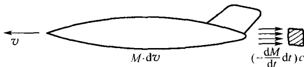
图 1.10 火箭在无外力作用下的运动
