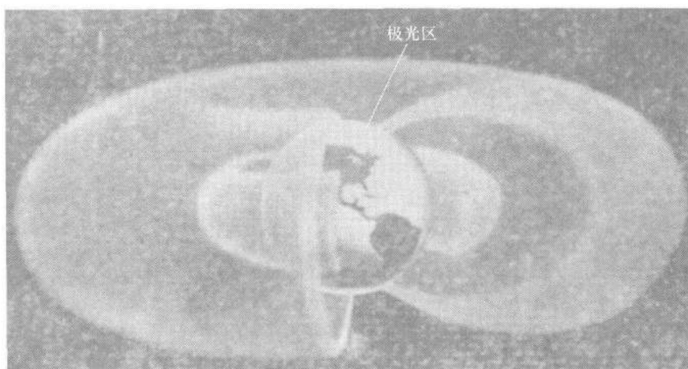
图 1.7 地球的内外辐射带
