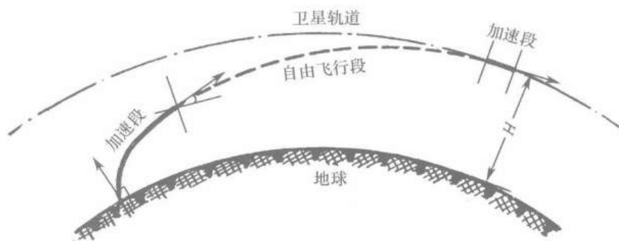
图 5.1 发射卫星的合理轨道
