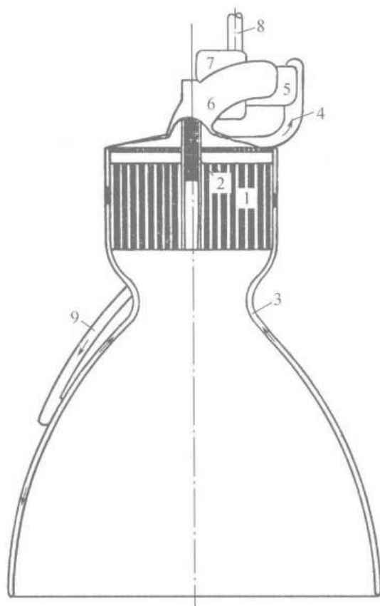
图 7.1 原子火箭发动机
