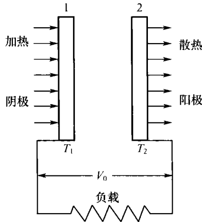
图 13.14 二极管热电子发电机原理图
