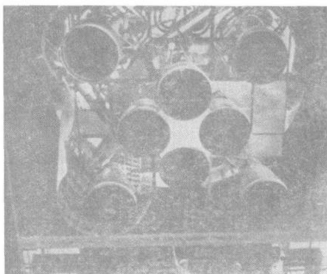
图 4.6 “土星”火箭第一级发动机的配置
