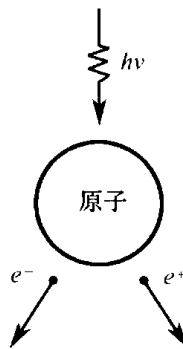
图 11.3 电子对的形成
