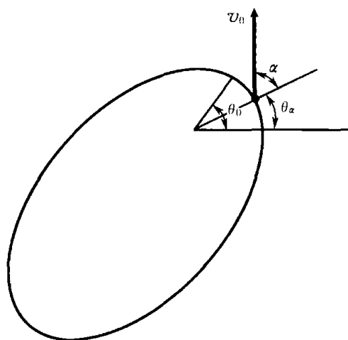
图 5.5 椭圆卫星轨道
