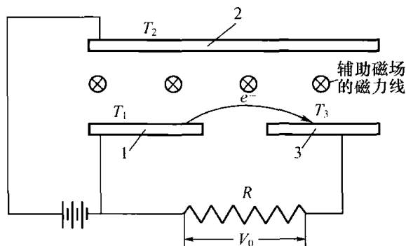
图 13.16 磁三极管热电子发电机原理图
